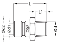
Plugs / Nippel
