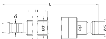
Plug / Nippel
