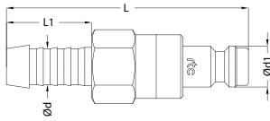
Plug / Nippel
